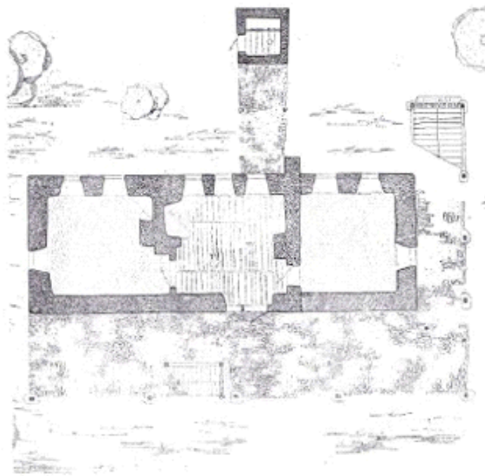
Casa aga Regep - plan etaj și fațadă
